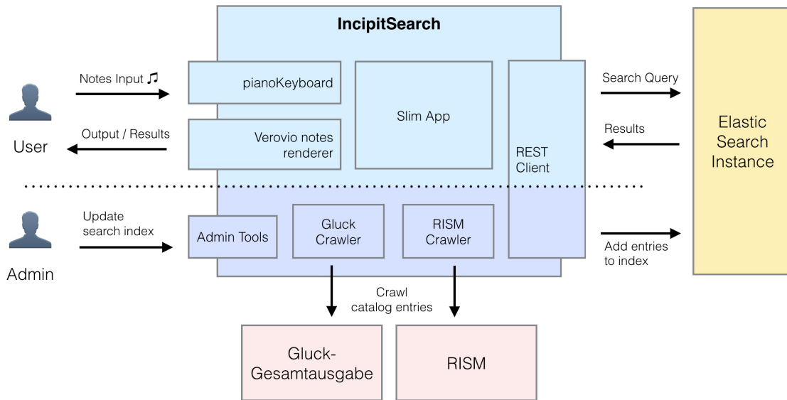
Abb. 1: Systemarchitektur der Incipit-Suche im Gluck-Werkverzeichnis.
